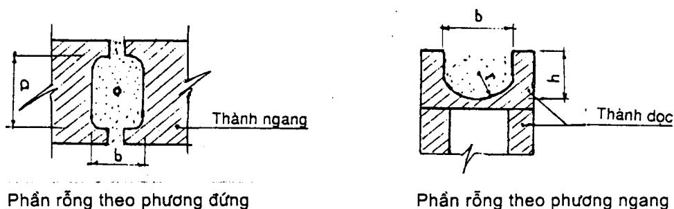
Hình 2 - Kích thước phần rỗng đặt cốt thép
